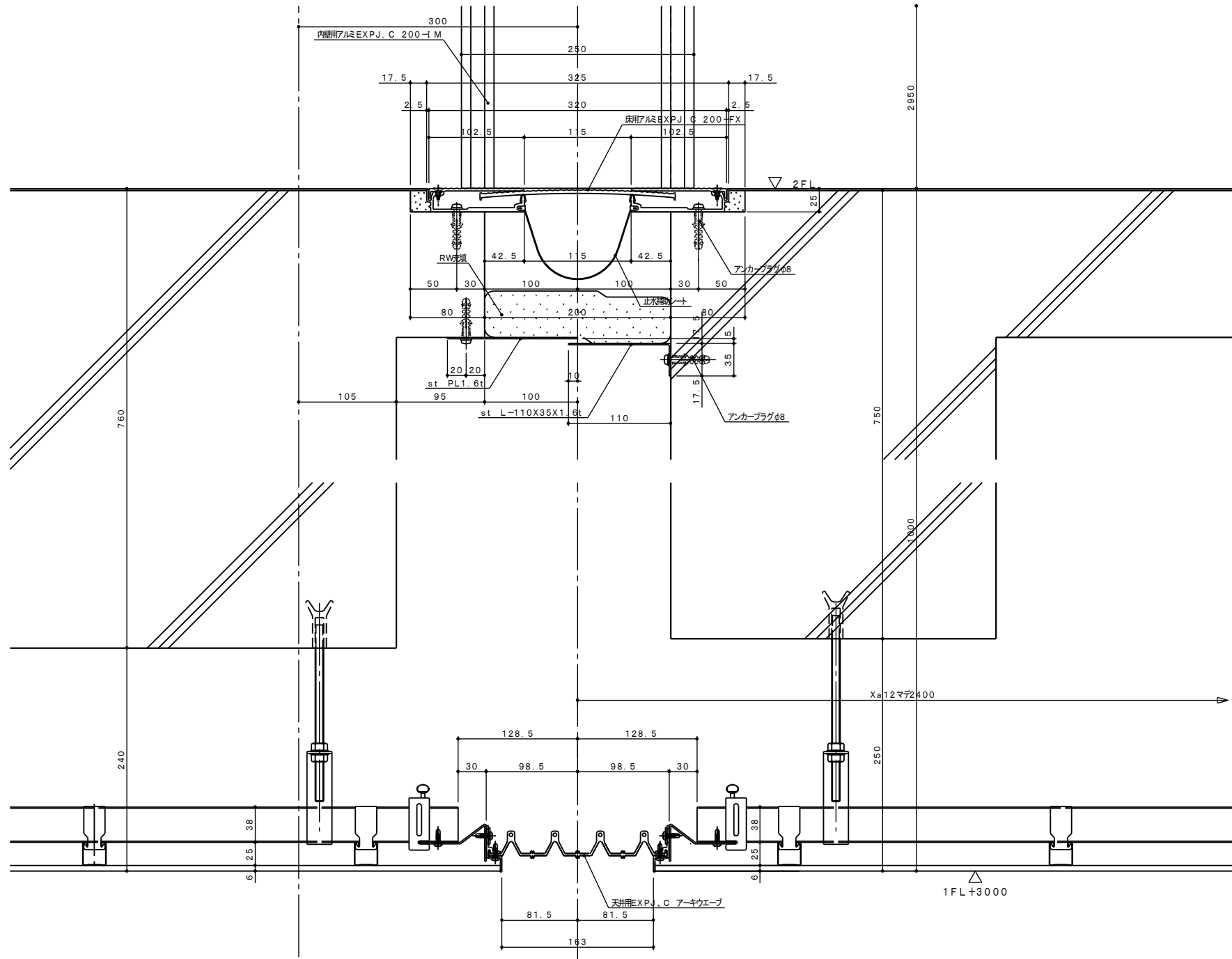
渡り廊下天井床用EXPJ. C断面詳細図 S: 1/2
