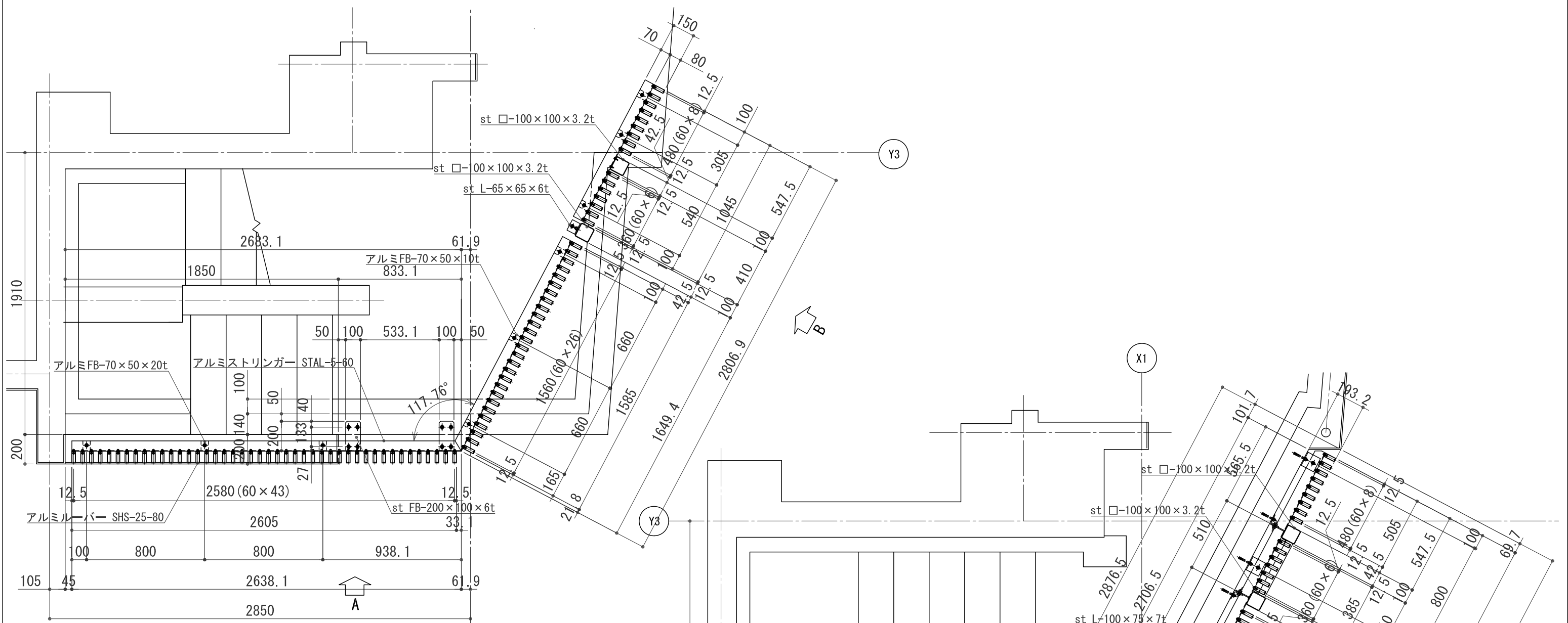
2F ルーバー 平面図 S:1/15
