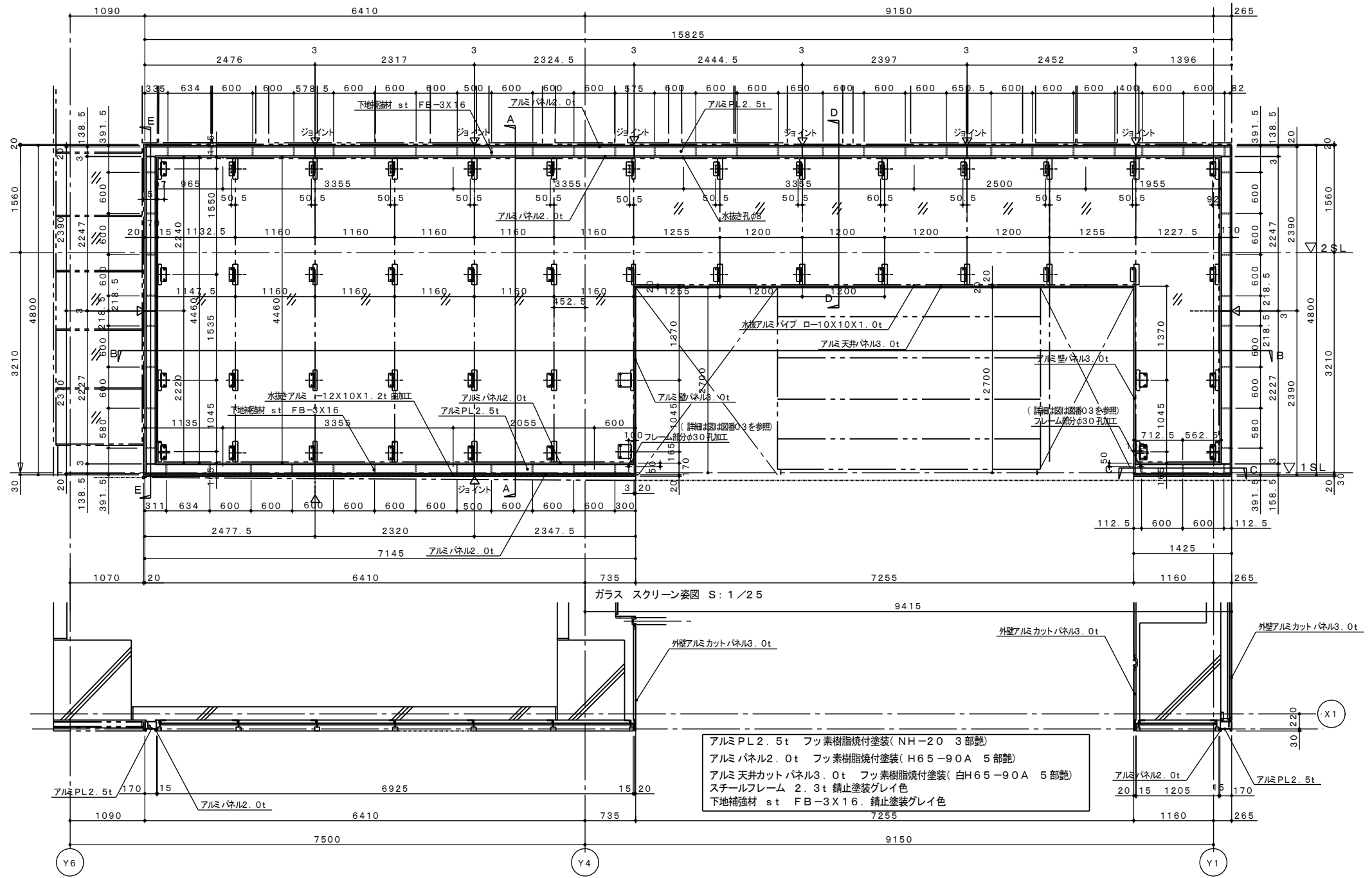
1F2Fガラス スクリーン 平面図 S: 1/25
