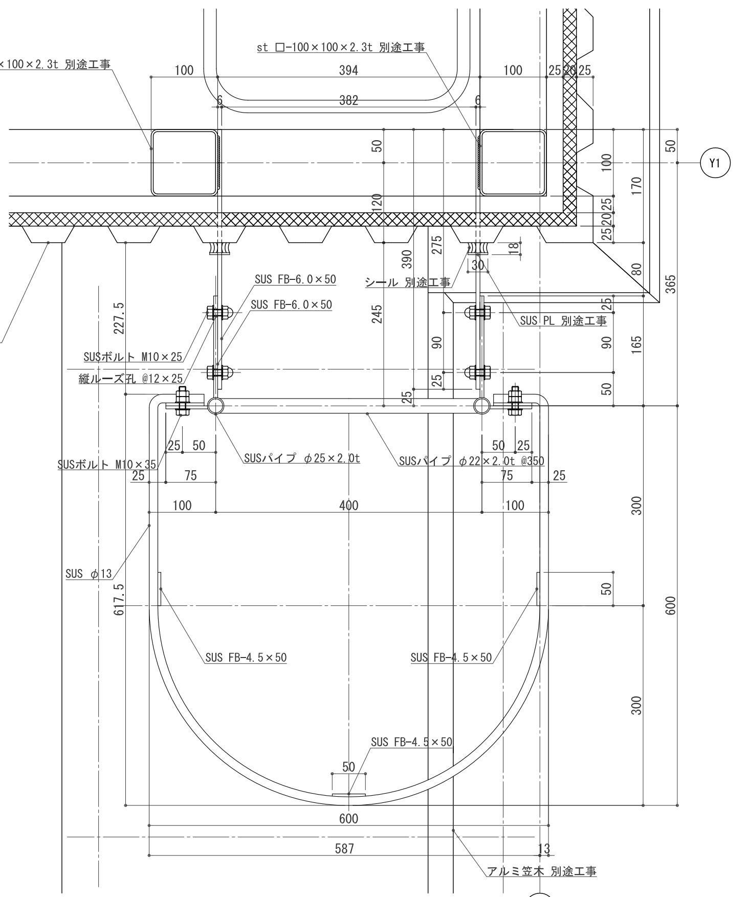
3F タラップ平面詳細図 S:1/3
