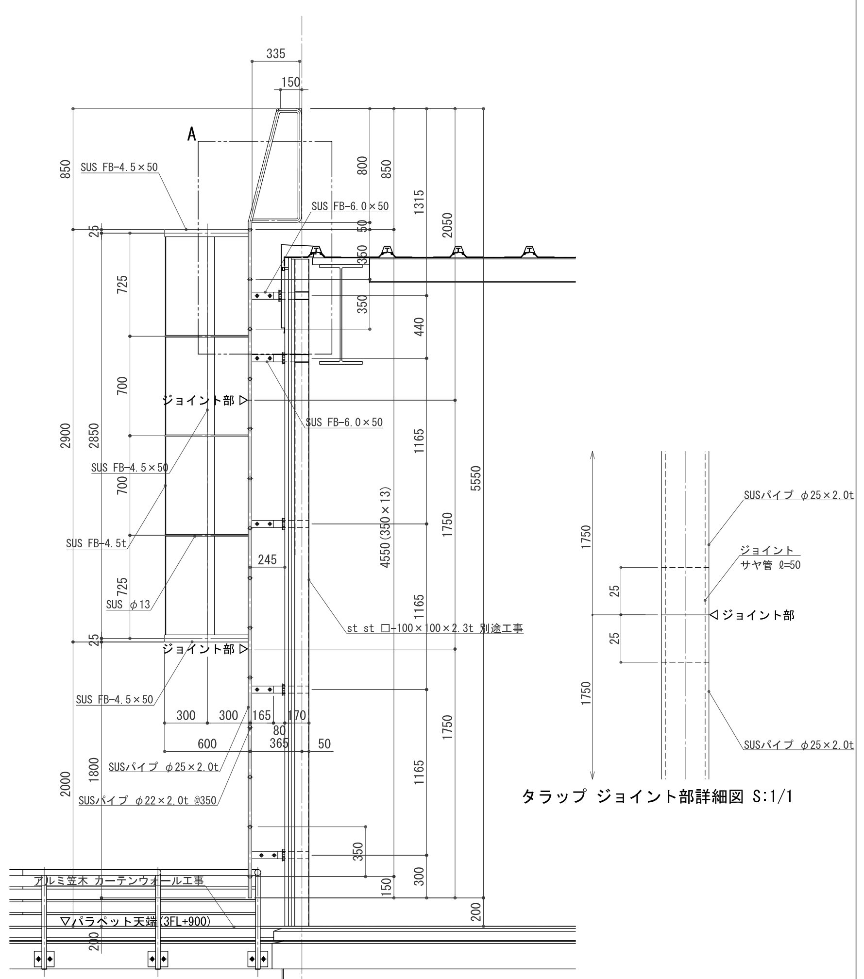
3F タラップ断面図 S:1/15 (Y1)
