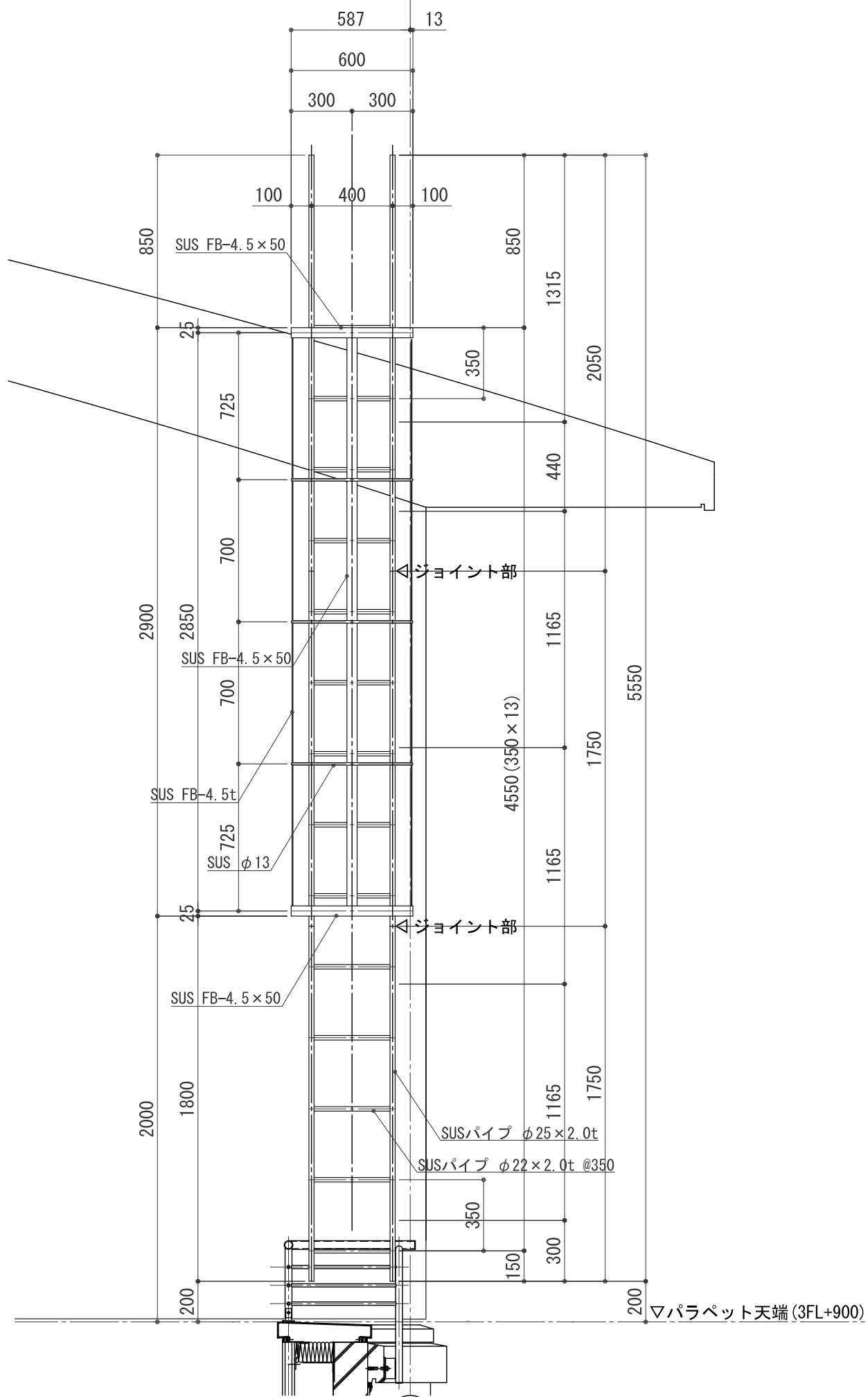
3F タラップ姿図 S:1/15 (X3)
