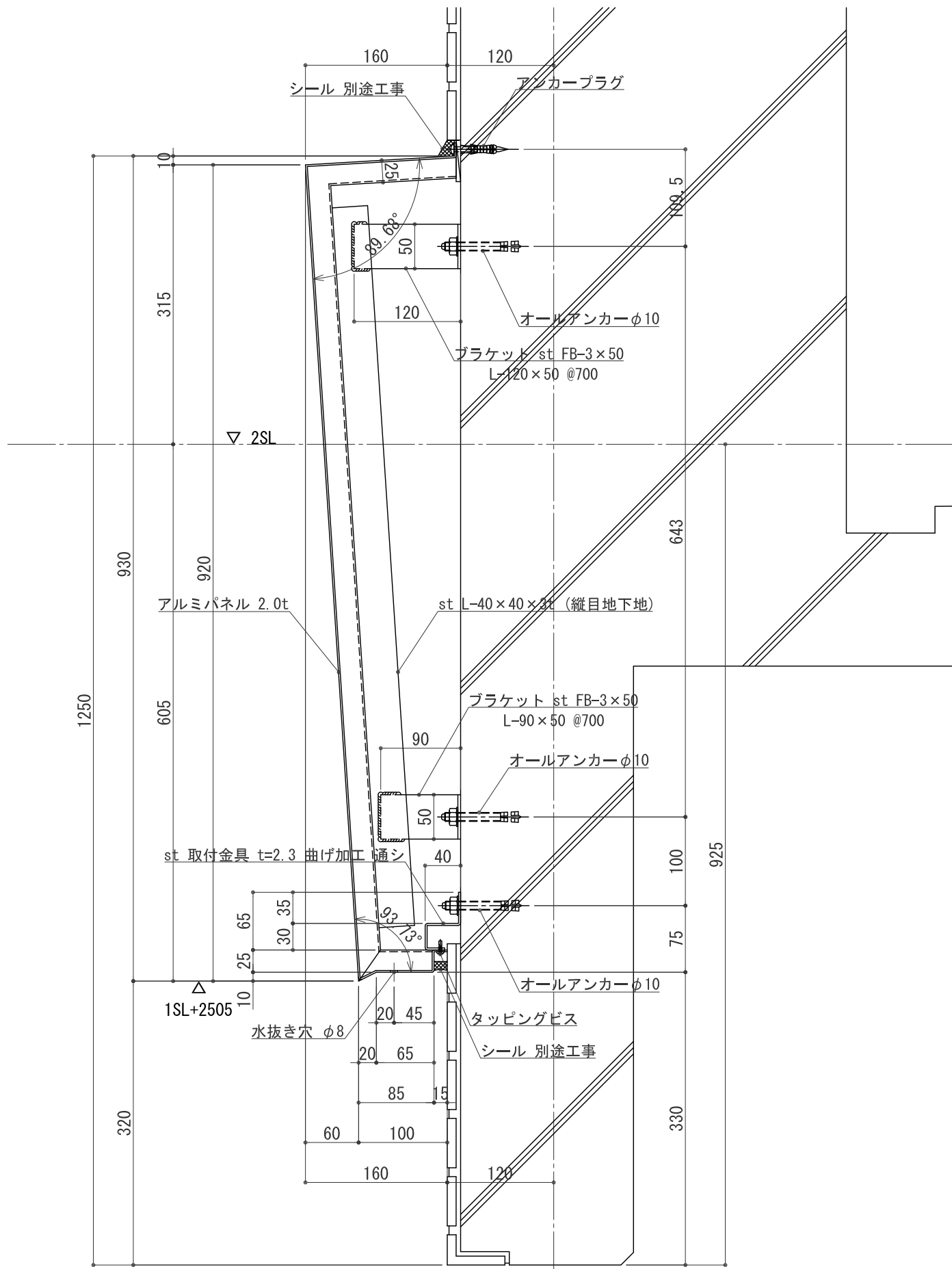
D断面詳細図 S:1/2 (X4)
