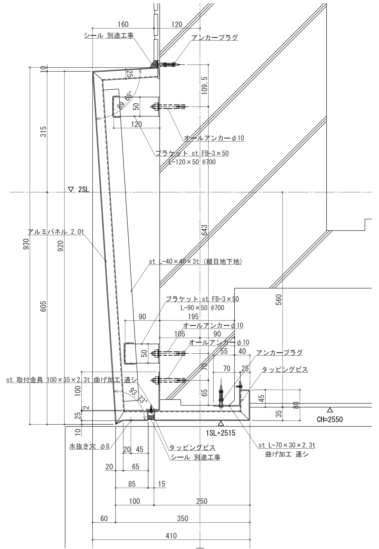
E断面詳細図 S:1/2 (X4)
