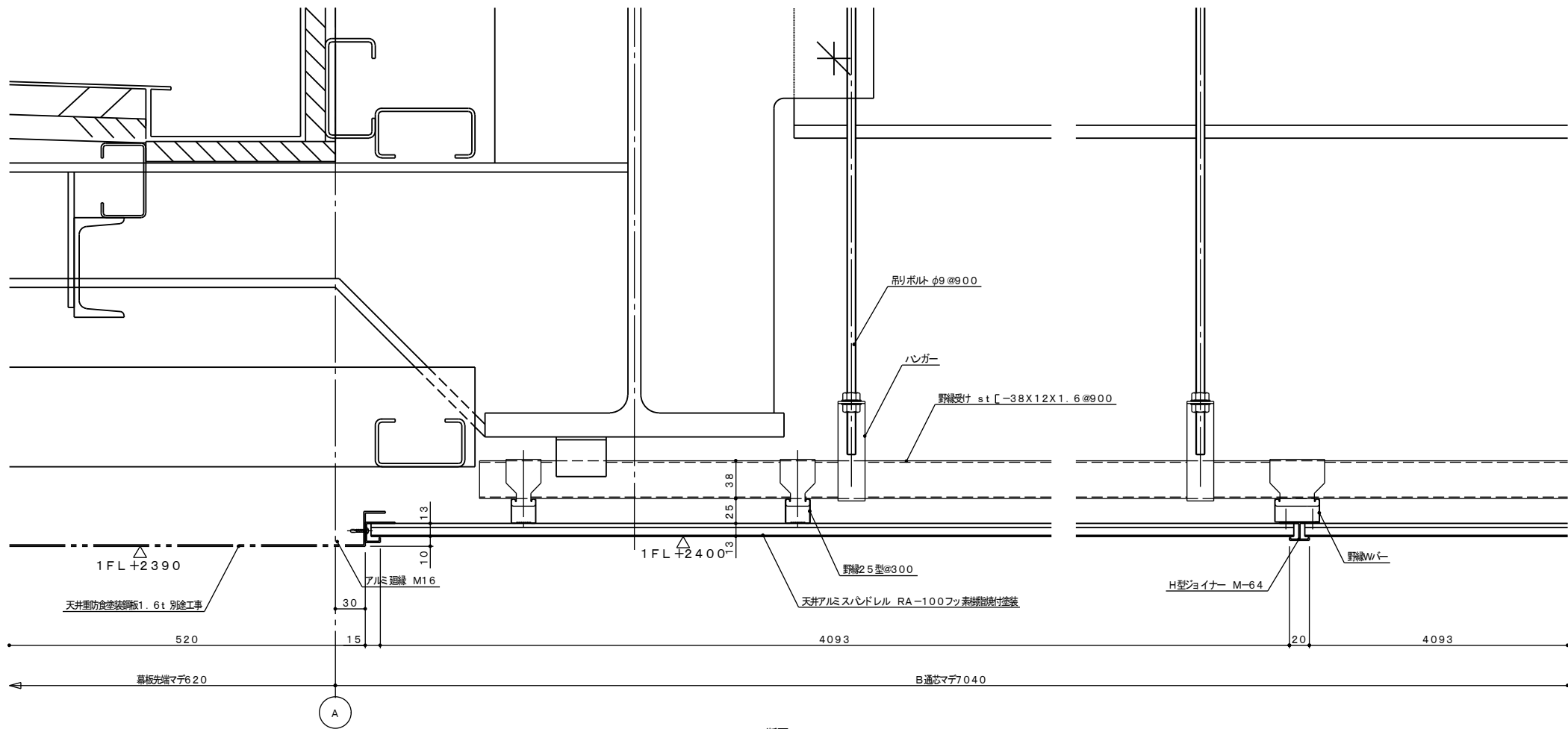
A 断面 駐車場天井断面詳細図 S : 1 / 2
