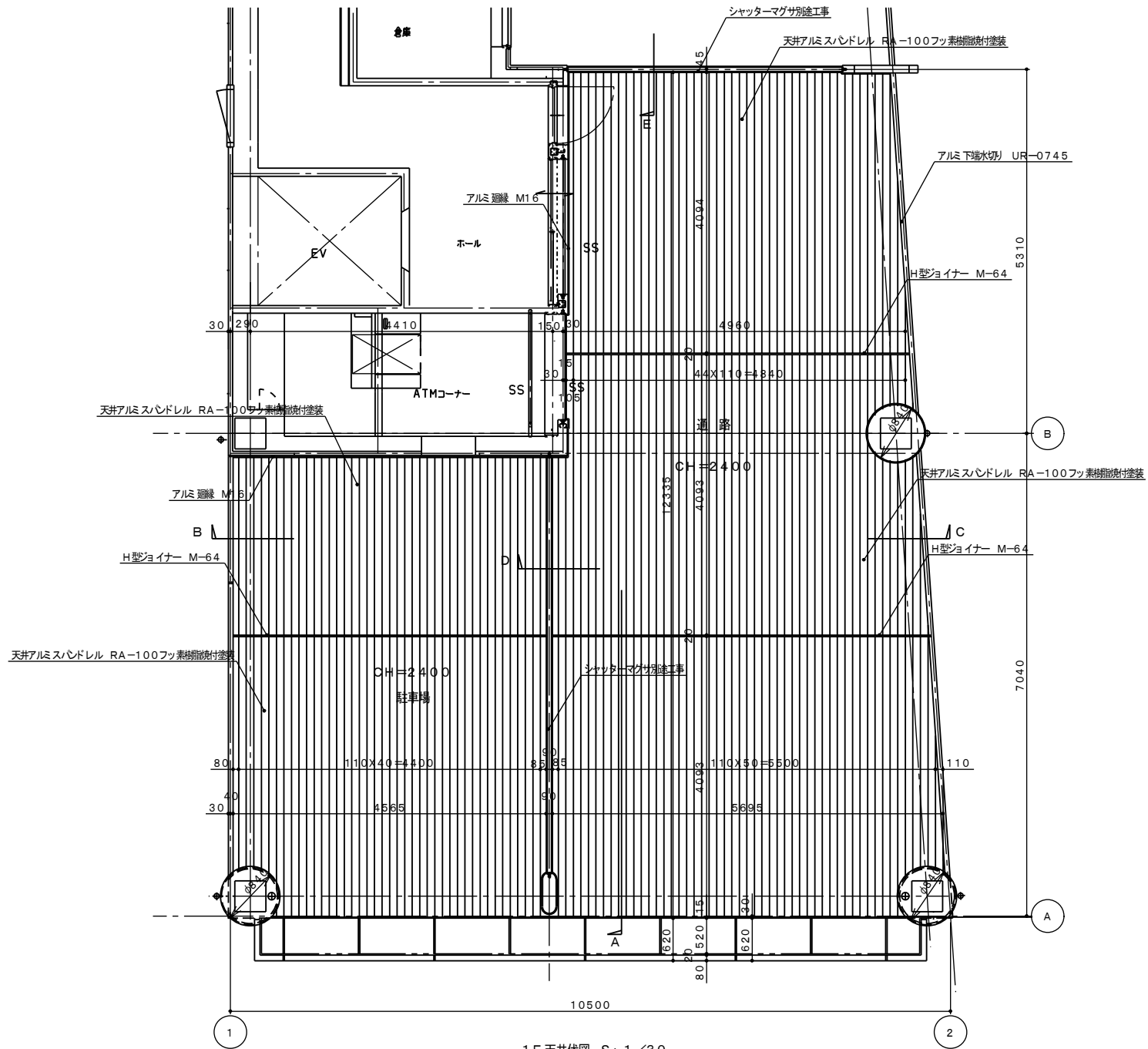
1F 天井伏図 S: 1/30
