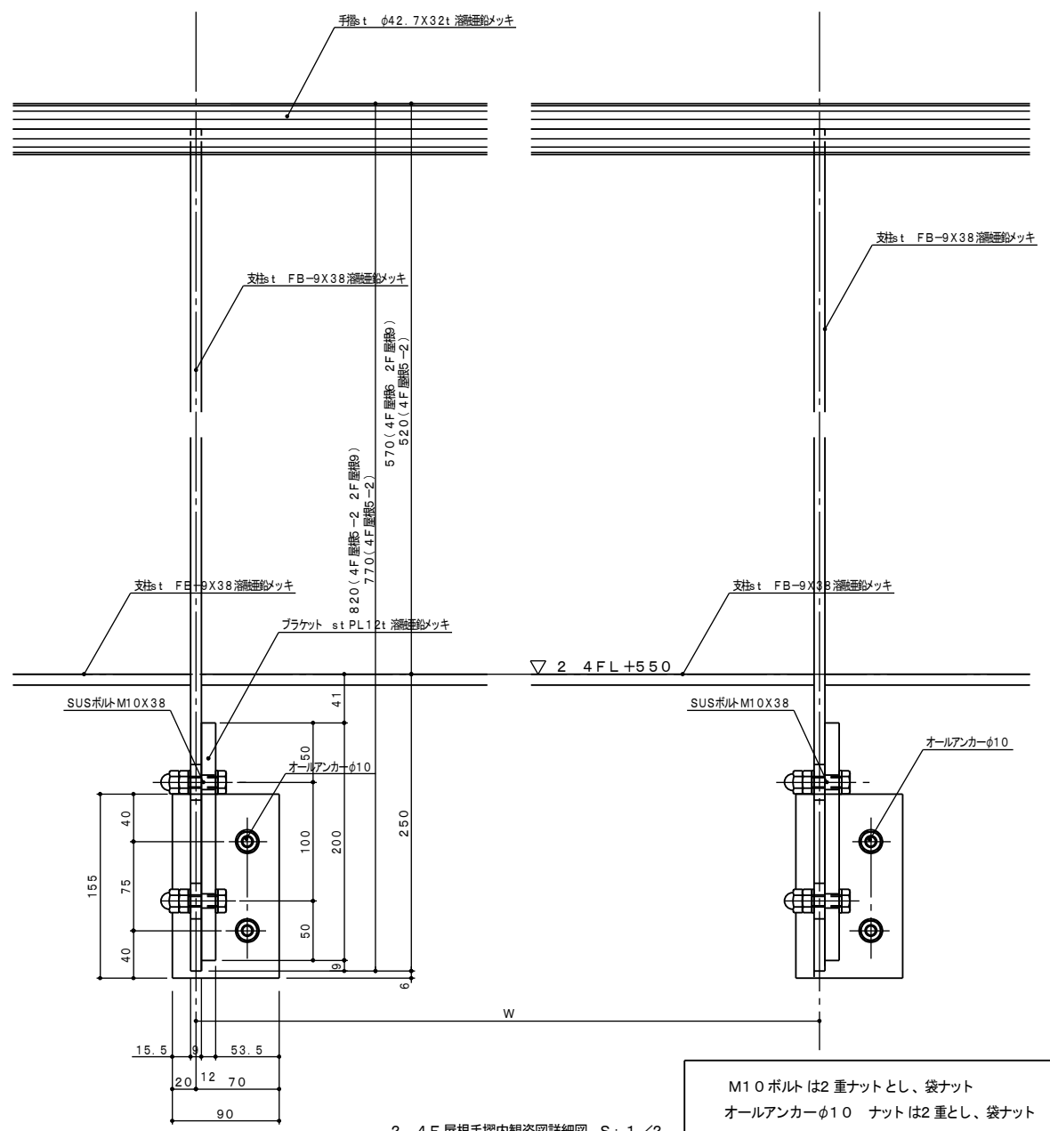
2 4F 屋根手摺内観姿図詳細図 S: 1/2
