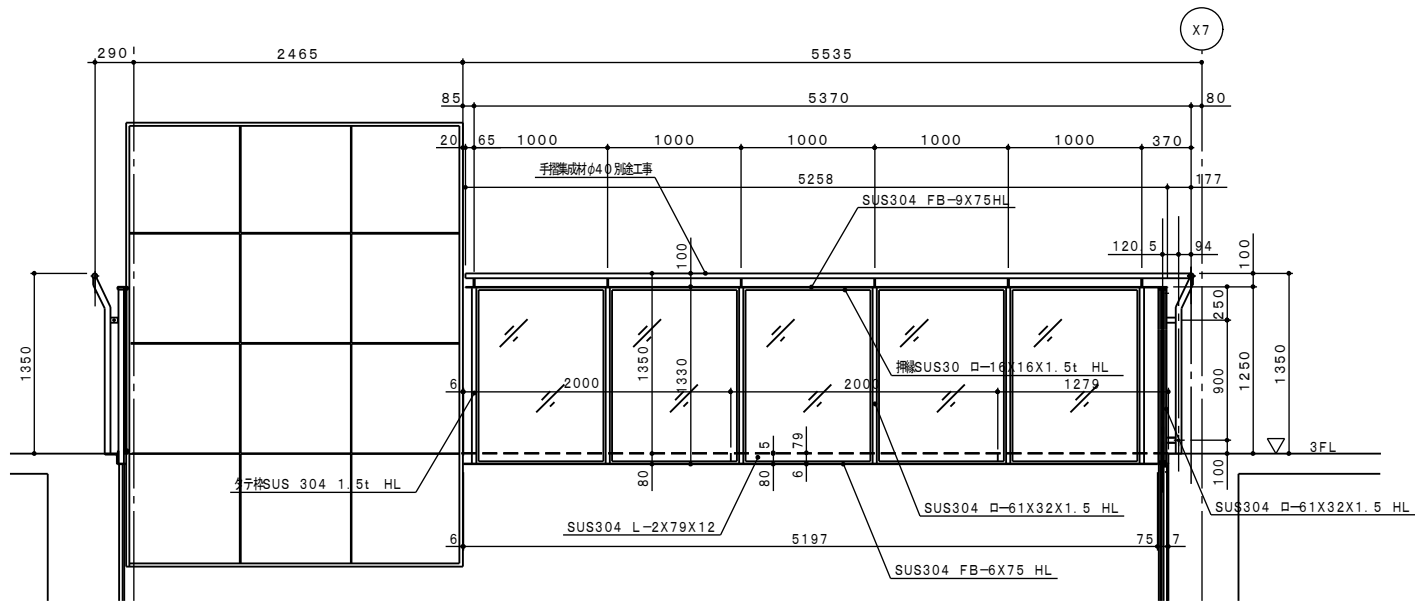
A 矢视图 S: 1/20
