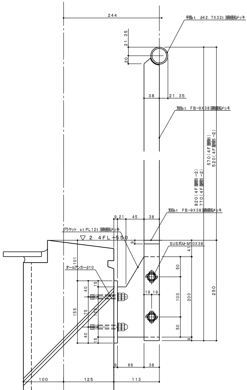
2 4F 屋根手摺断面詳細図 S: 1/2
