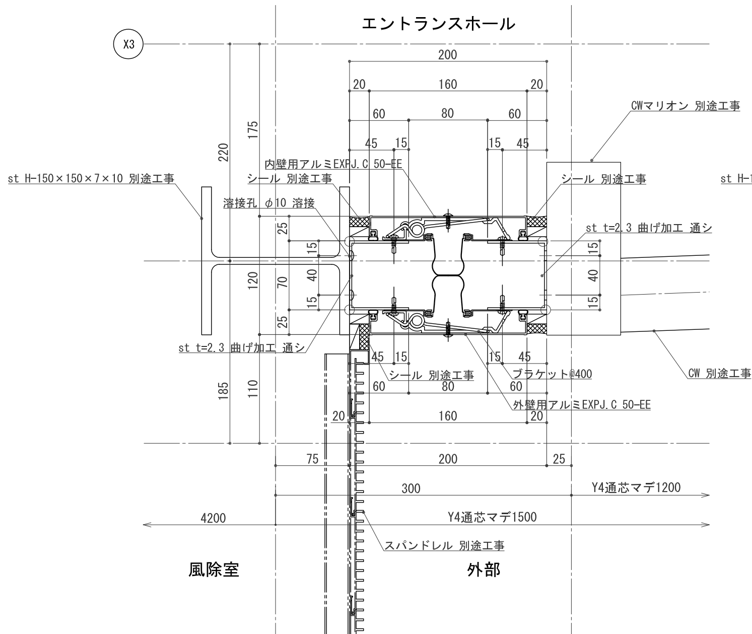
1F EXPJ.C 平面詳細図 S:1/2
