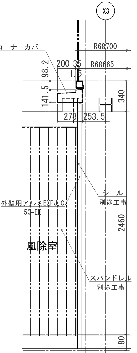
EXPJ.C 姿図 S:1/15
