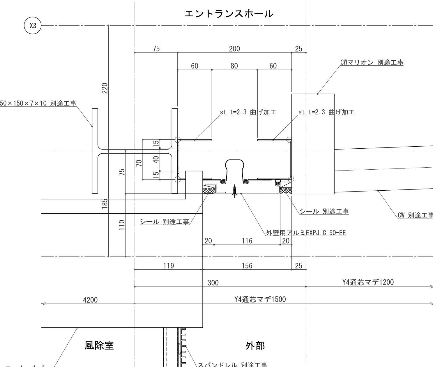
2F EXPJ.C 平面詳細図 S:1/2
