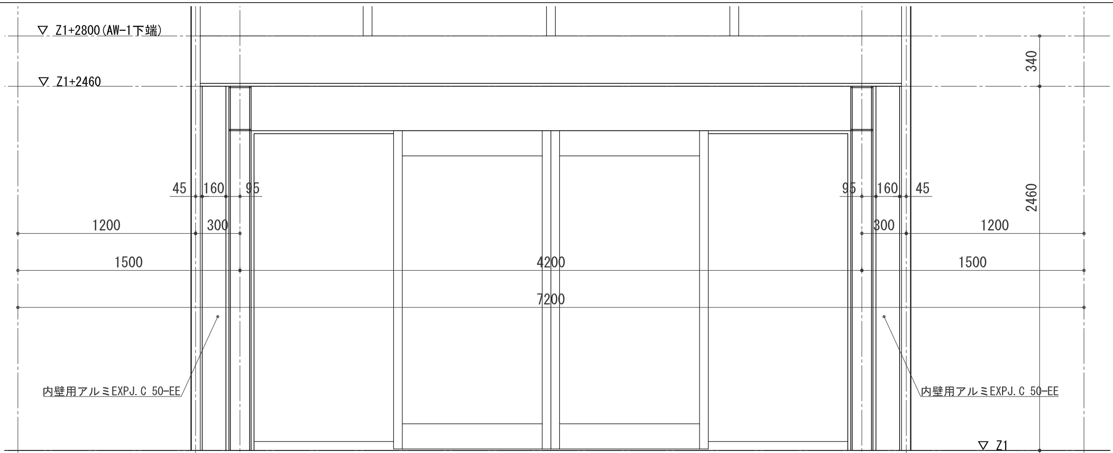
エントランス側ヨリ EXPJ.C 姿図 S:1/15
