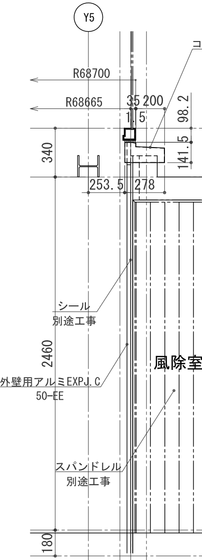
EXPJ.C 姿図 S:1/15
