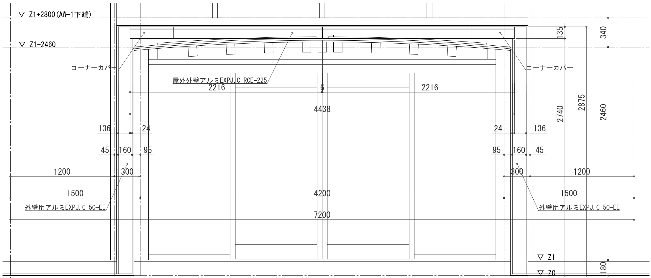
風除室側ヨリ EXPJ.C 姿図 S:1/15
