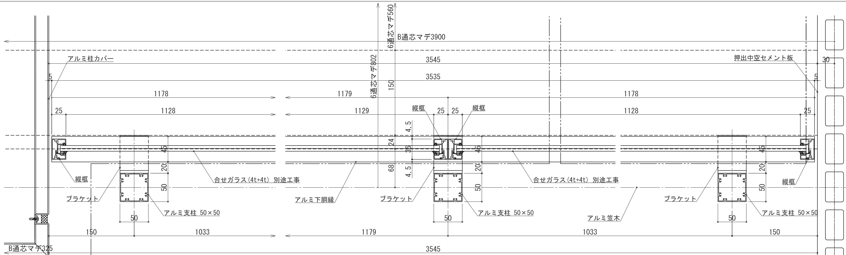
3F 壁付手摺 平面詳細図 S:1/2
