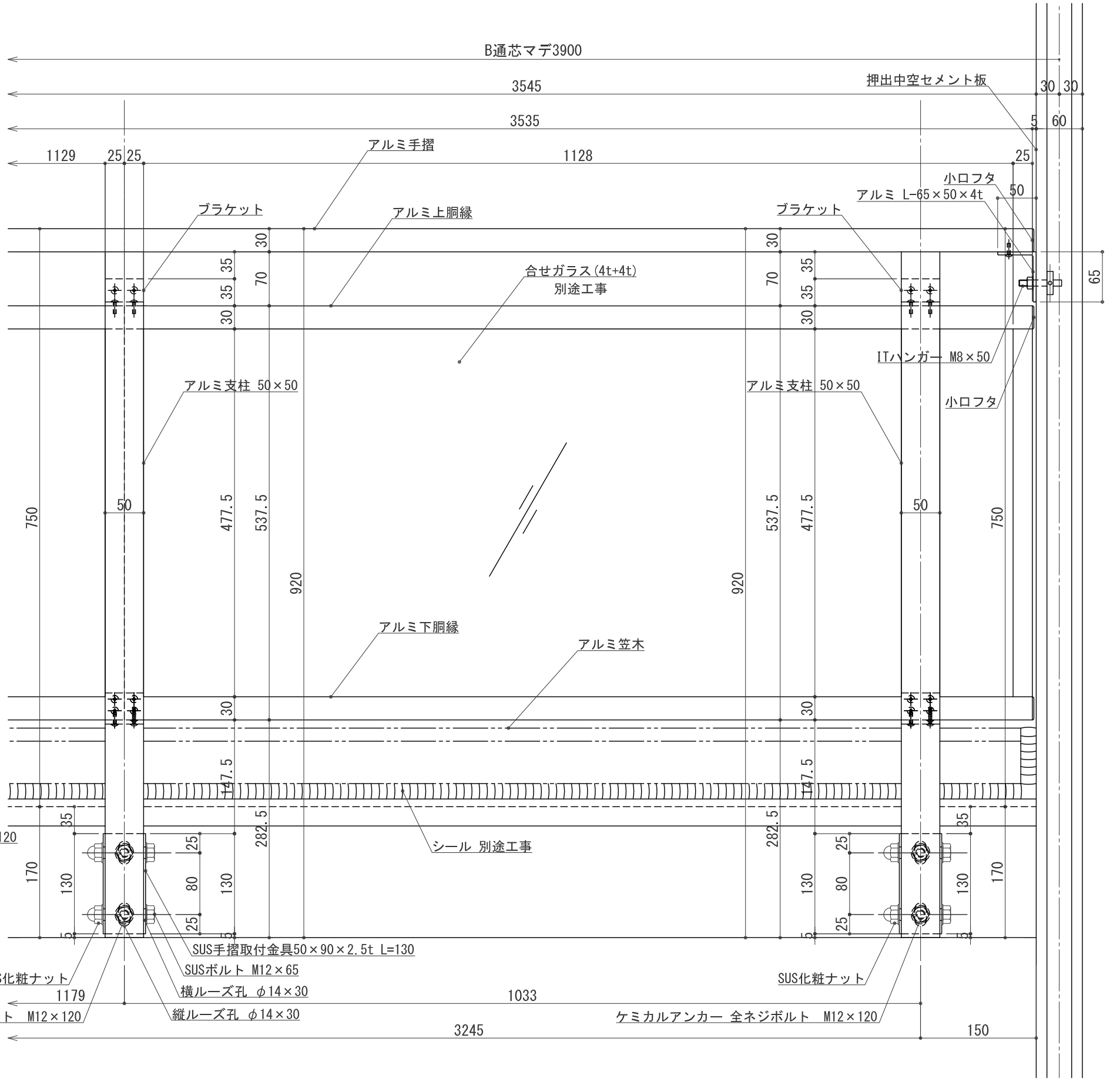
3F 壁付手摺 姿図詳細図 S:1/3
