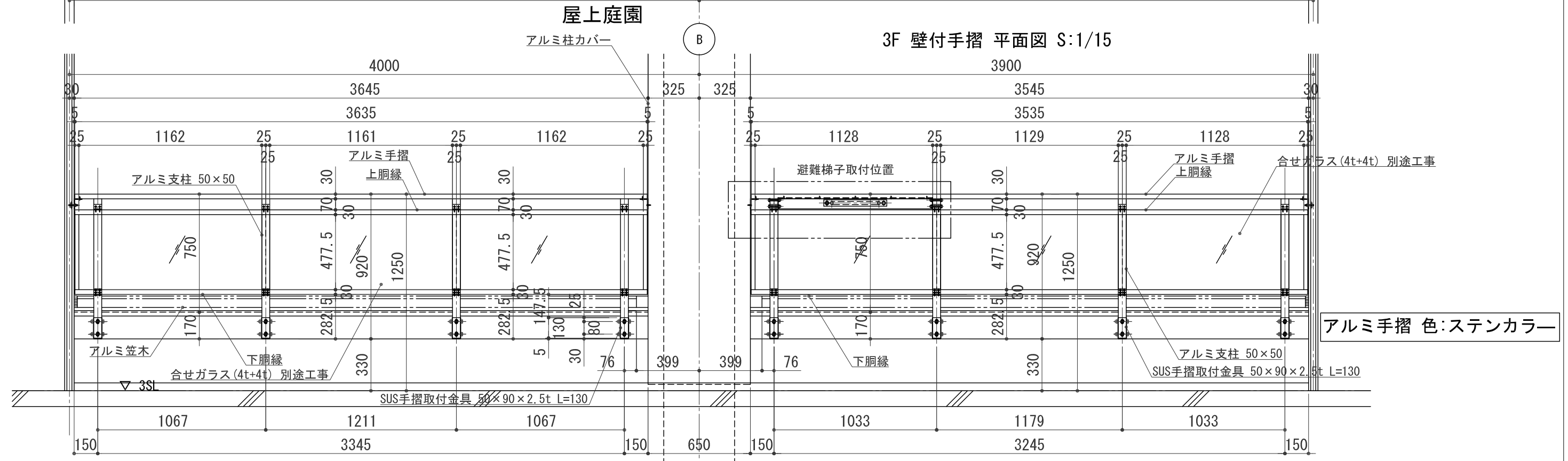
3F 壁付手摺 姿図 S:1/15
