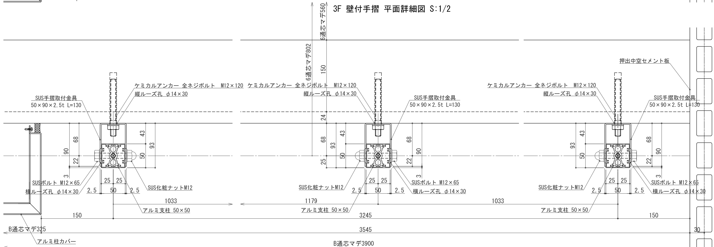
3F 壁付手摺 平面詳細図 S:1/2
