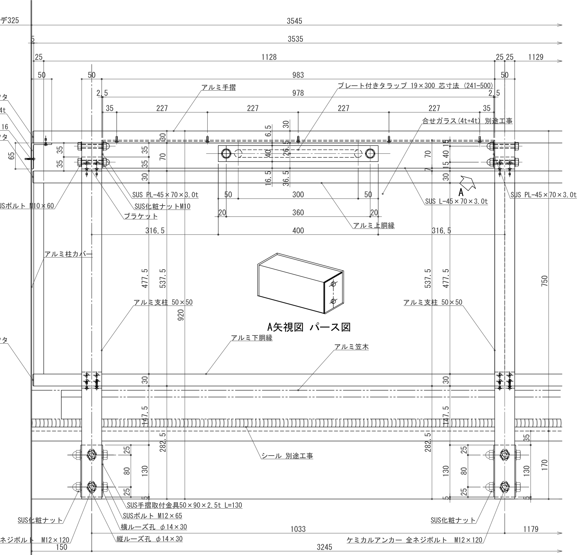
3F 避難梯子取付部 アルミ手摺 姿図詳細図 S:1/3
