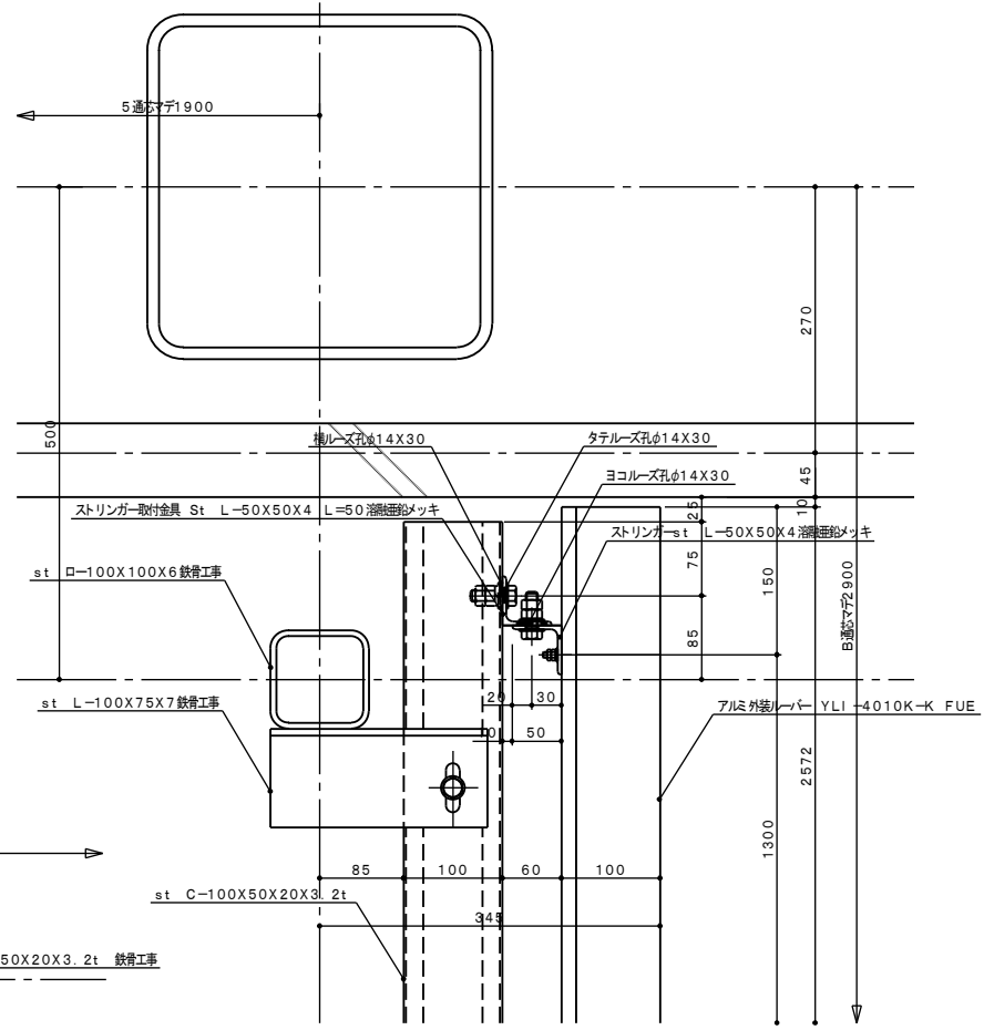
R 部詳細図 S: 1/3
