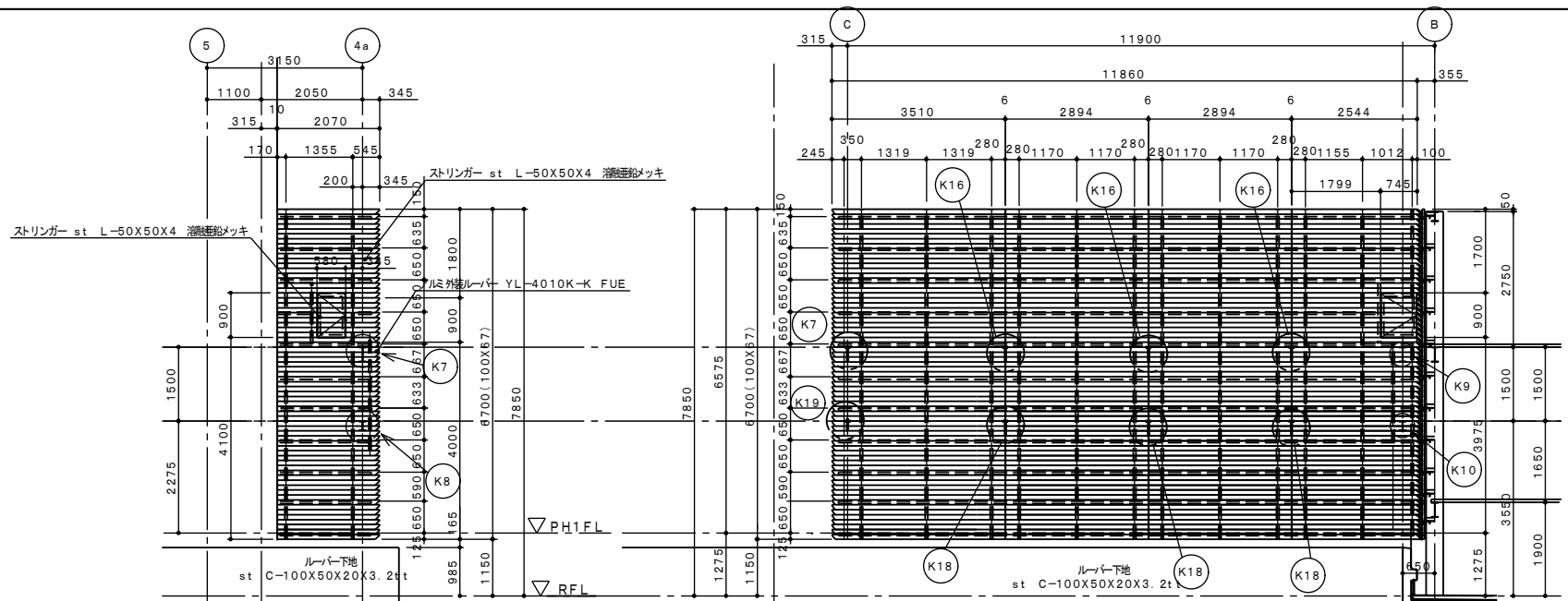
カ矢視 外装ルーバー姿図 S: 1/50
