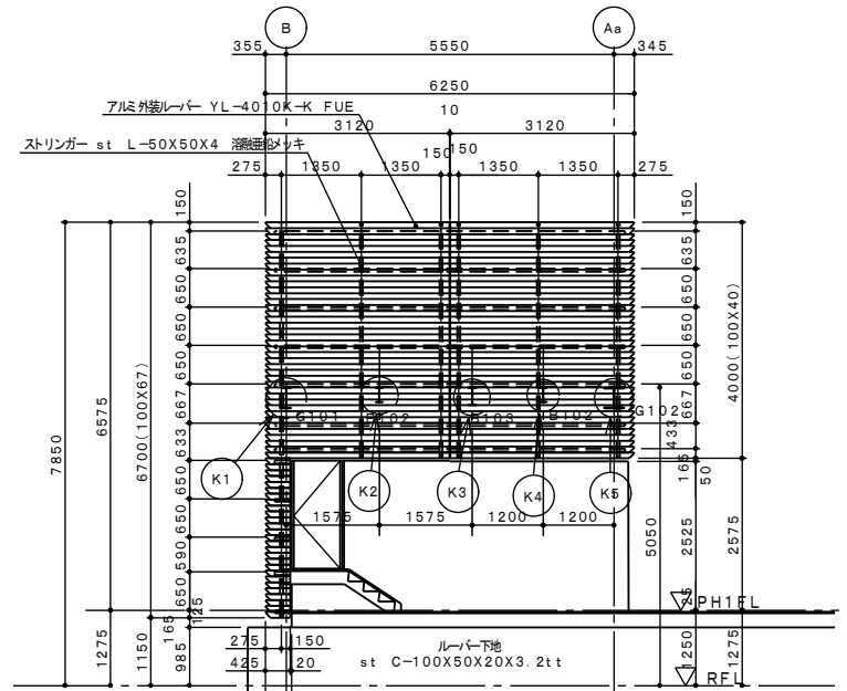
バ矢視 外装ルーバー姿図 S: 1/50
