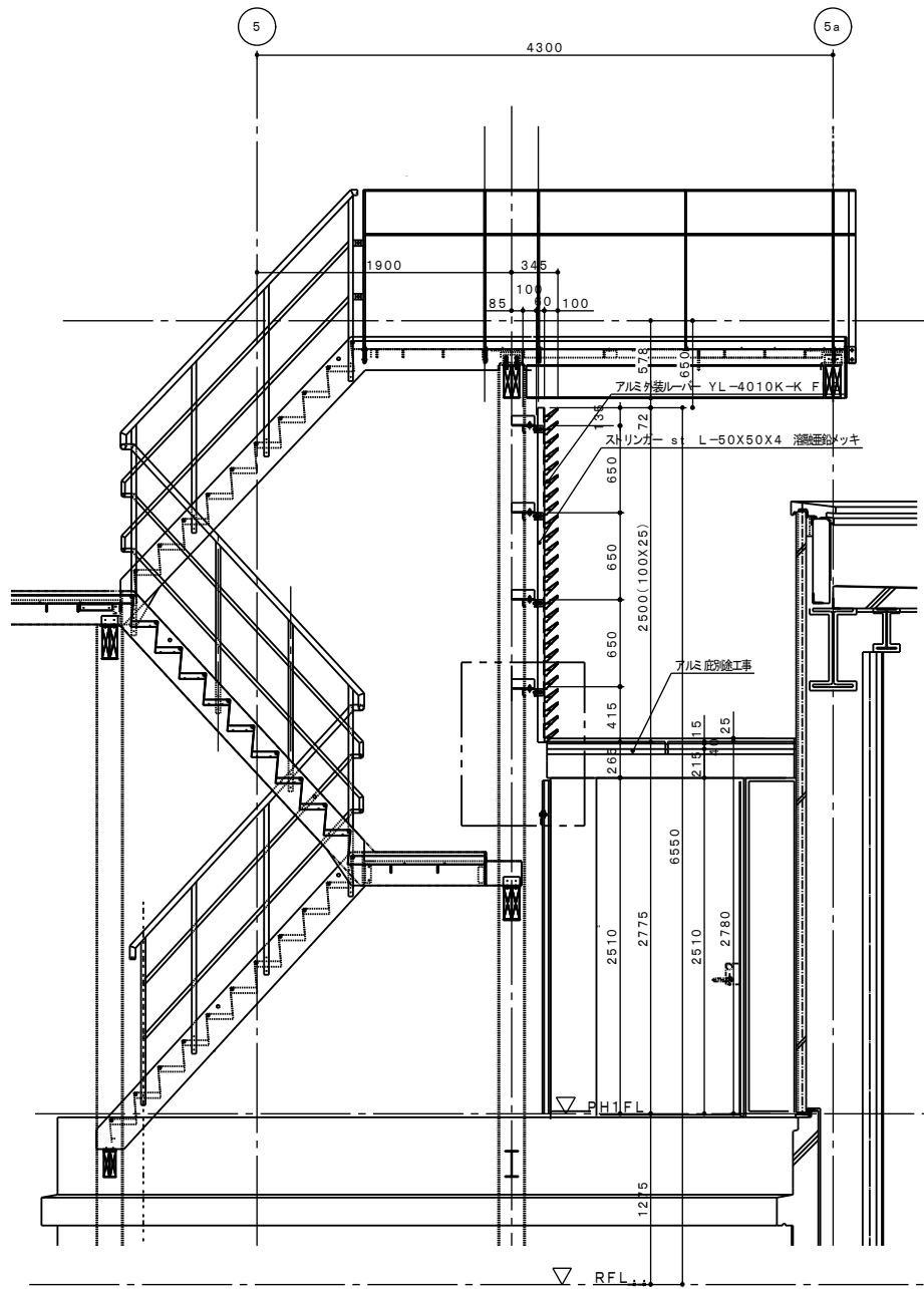
H~H断面 S: 1/20
