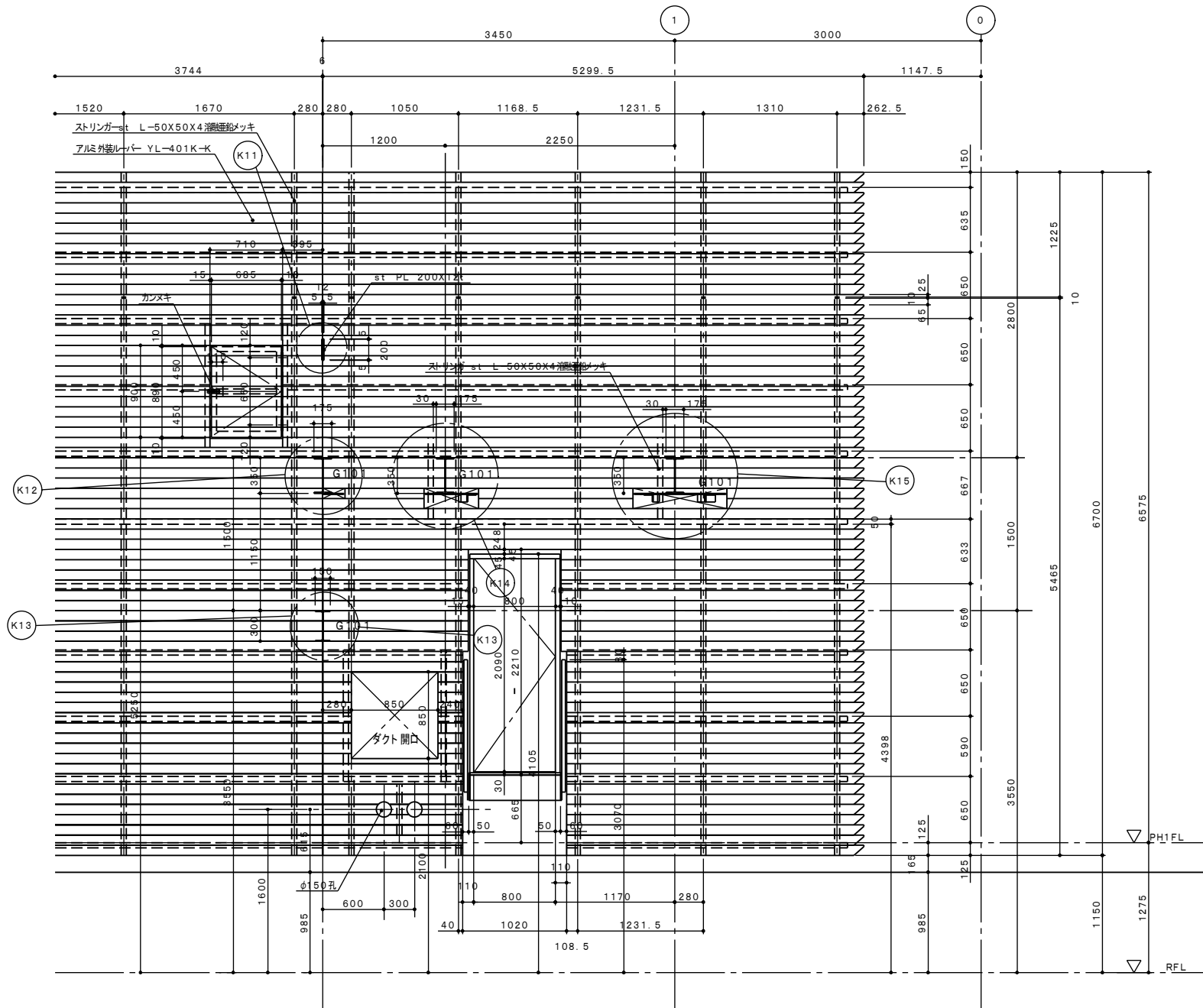
工矢視図部分姿図詳細図 S: 1 / 20
