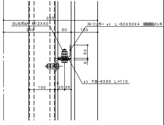
ストリンガージョイント部断面詳細図 S: 1/3
