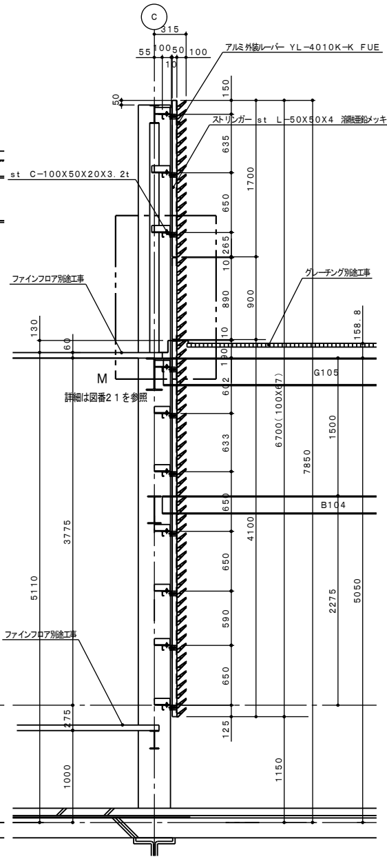
E~E断面 S: 1/20
