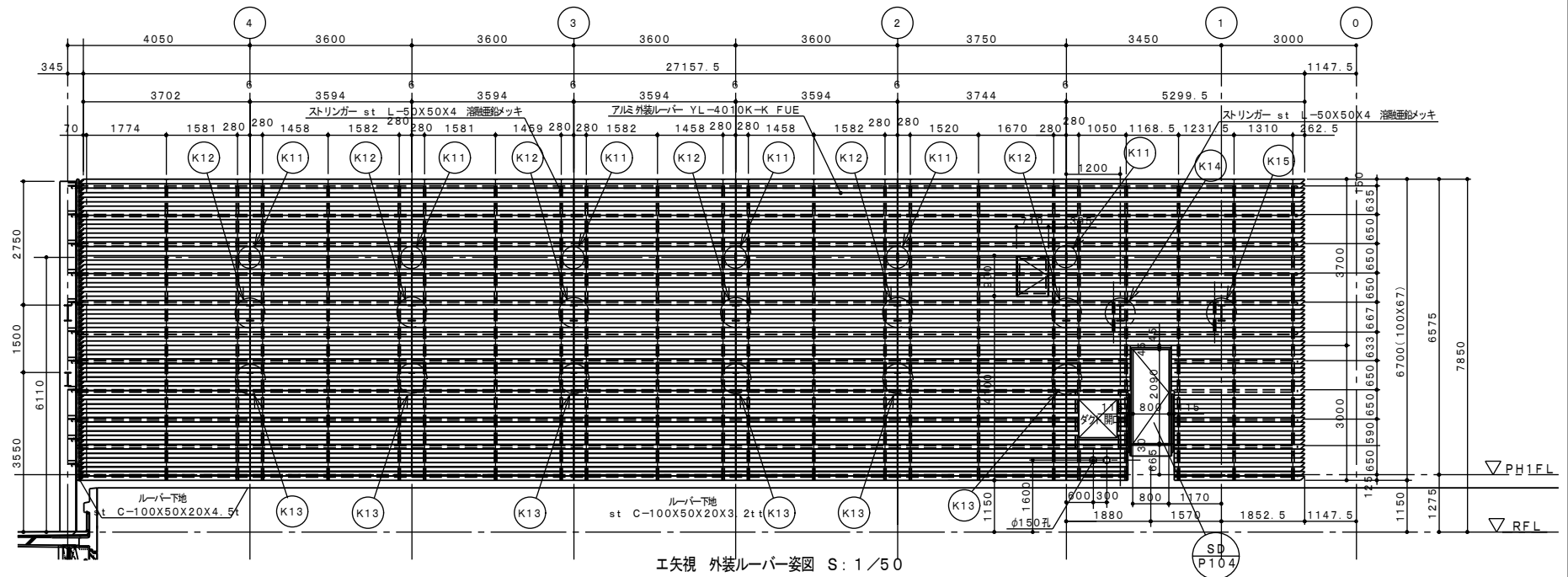
カ矢視 外装ルーバー姿図 S: 1/50
