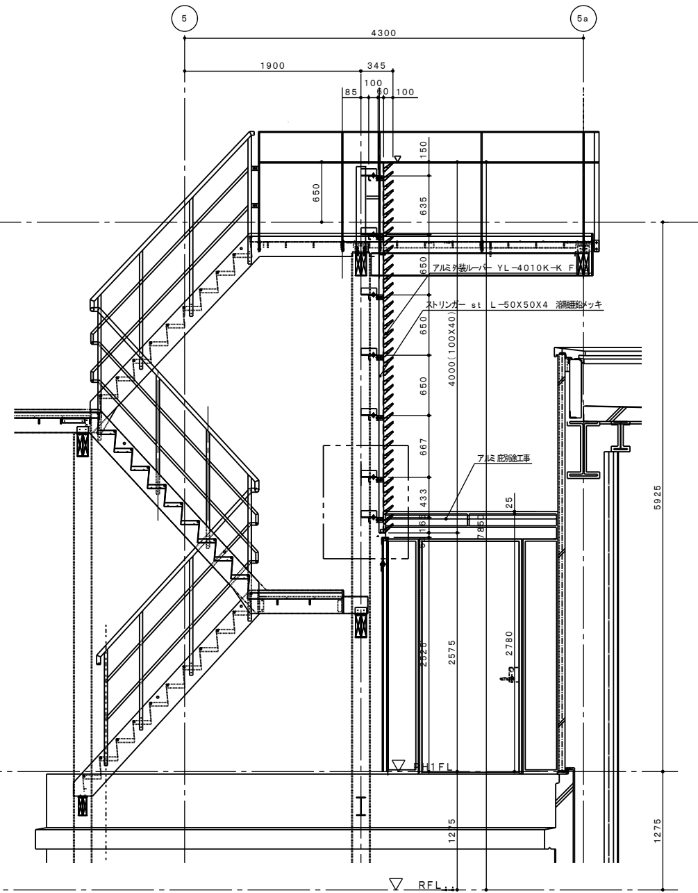
G~G断面 S: 1/20
