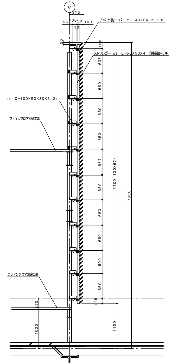
F~F断面 S: 1/20
