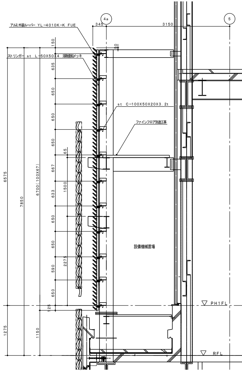
D~D断面 S: 1/20
