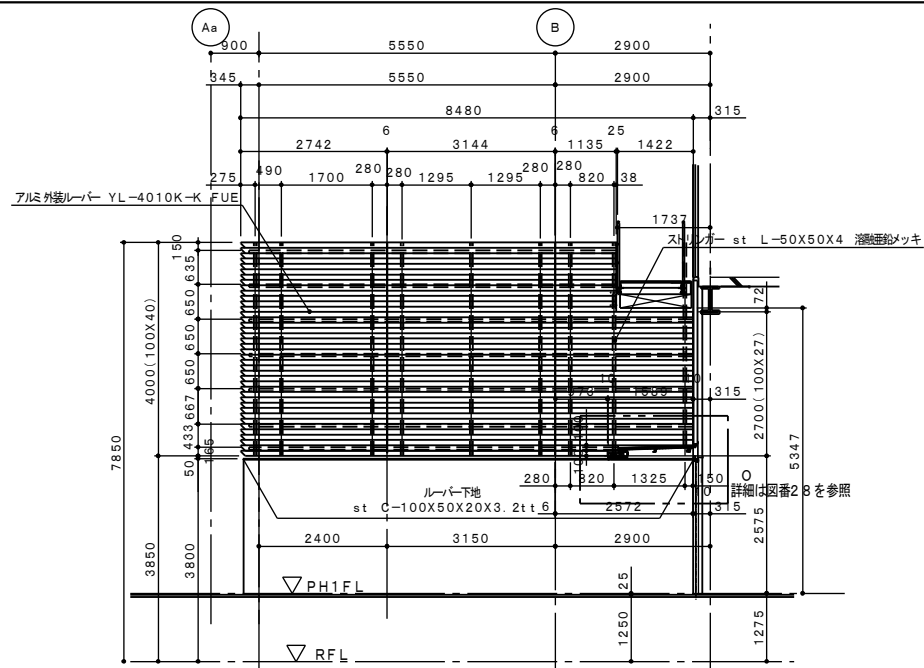
ア矢視 外装ルーバー姿図 S: 1/50
