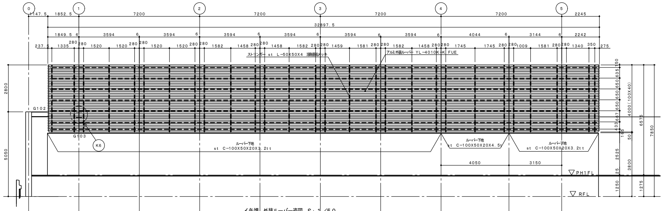
イ矢視 外装ルーバー姿図 S: 1/50
